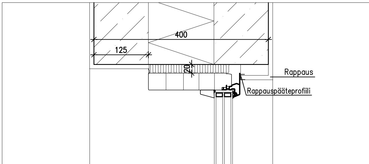
DET 2A 1:5 (Ikkunan yläreuna)
