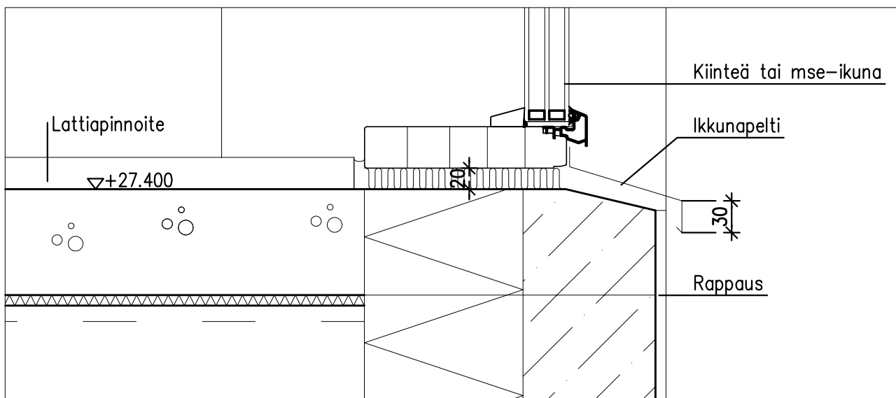
DET 2C 1:5 (Ikkunan alareuna)
