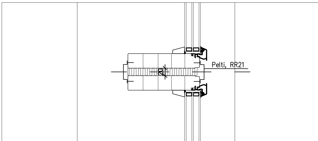
DET 2B 1:5 (päällekkäisten ikkunoiden liitos)
