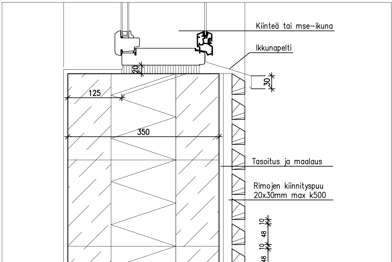
DET 3A 1:5 (rimotus julkisivussa, pystyleikkaus)
