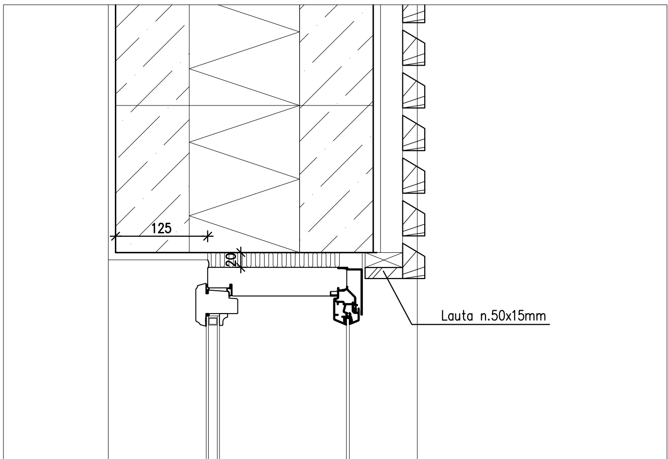
DET 3B 1:5 (rimotus julkisivussa, pystyleikkaus)
