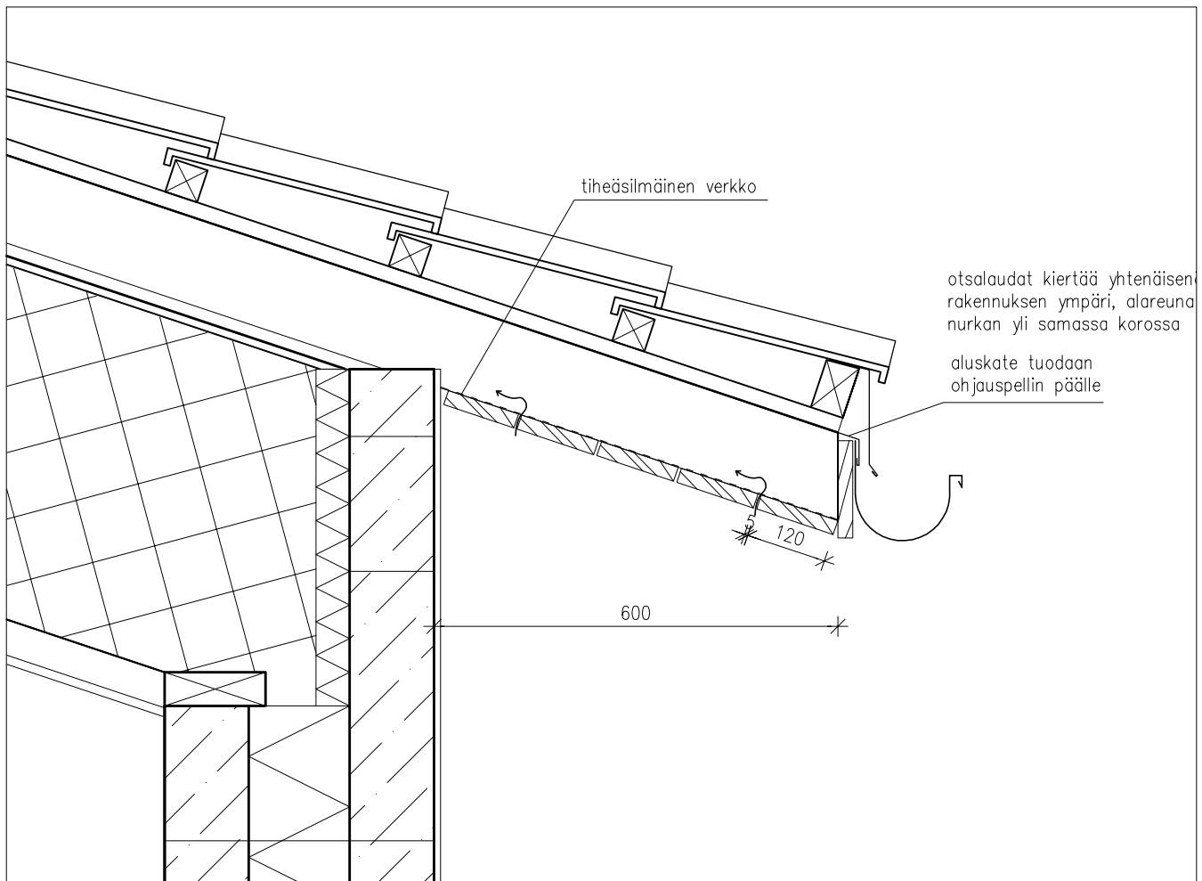
DET R1 1:10 (alaräystäs)
