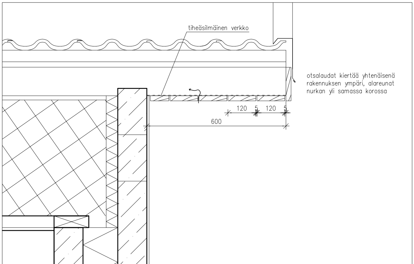
DET R2 1:10 (sivuräystäs)
